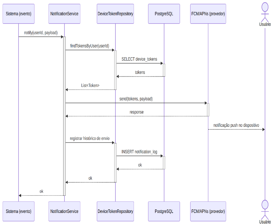
Figura 22 — Diagrama de sequência do UC22 (Receber notificações push).
