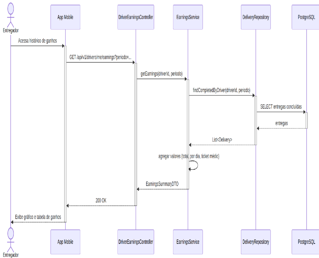
Figura 27 — Diagrama de sequência do UC27 (Consultar histórico de ganhos).
