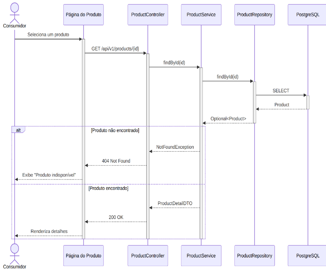
Figura 5 — Diagrama de sequência do UC05 (Visualizar detalhe do produto).
