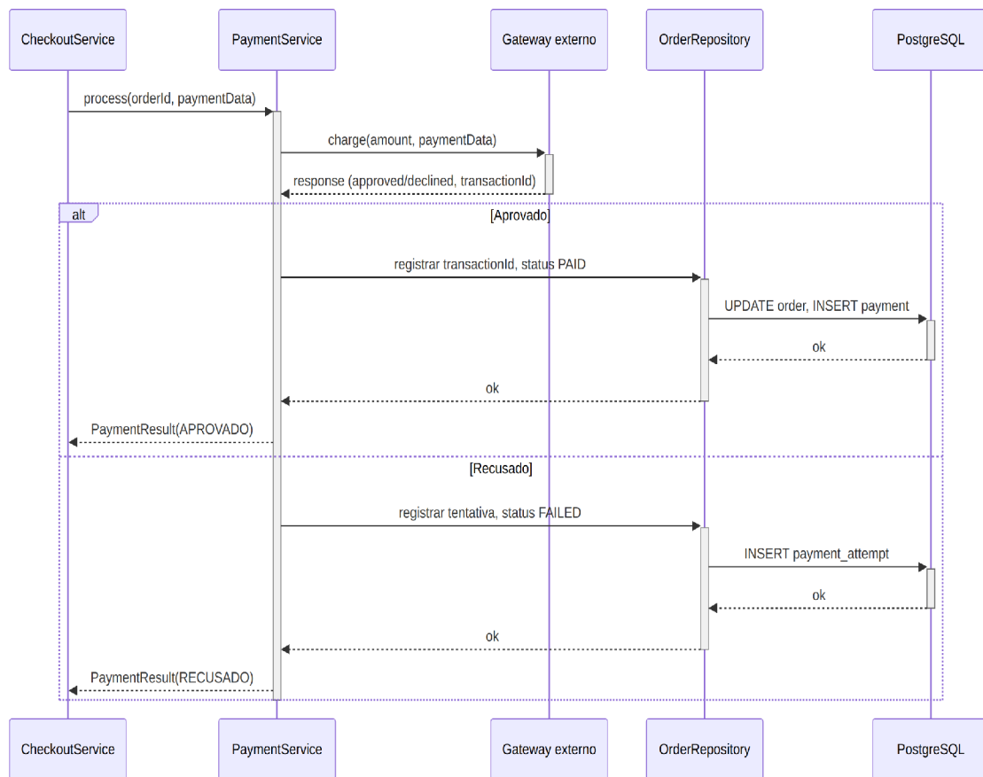
Figura 23 — Diagrama de sequência do UC23 (Gateway de pagamento).
