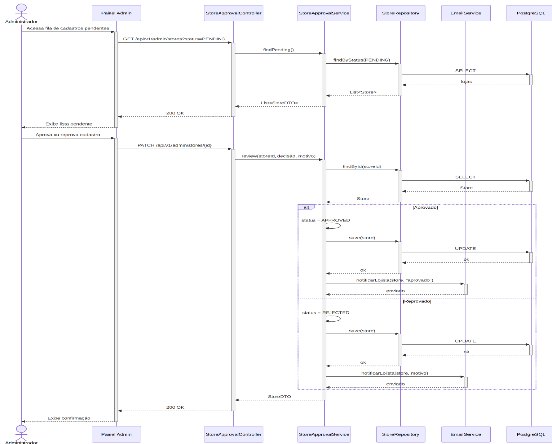
Figura 24 — Diagrama de sequência do UC24 (Aprovar ou reprová cadastro do lojista).
