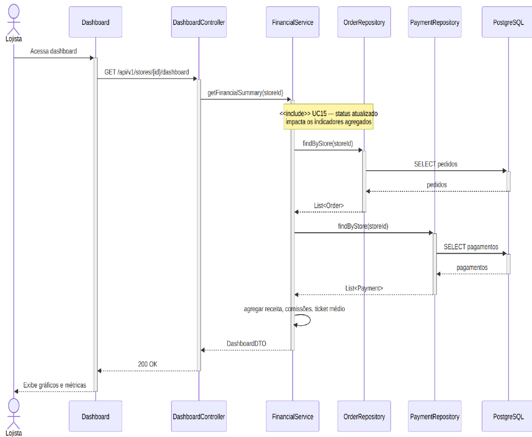
Figura 11 — Diagrama de sequência do UC11 (Visualizar dashboard financeiro).
