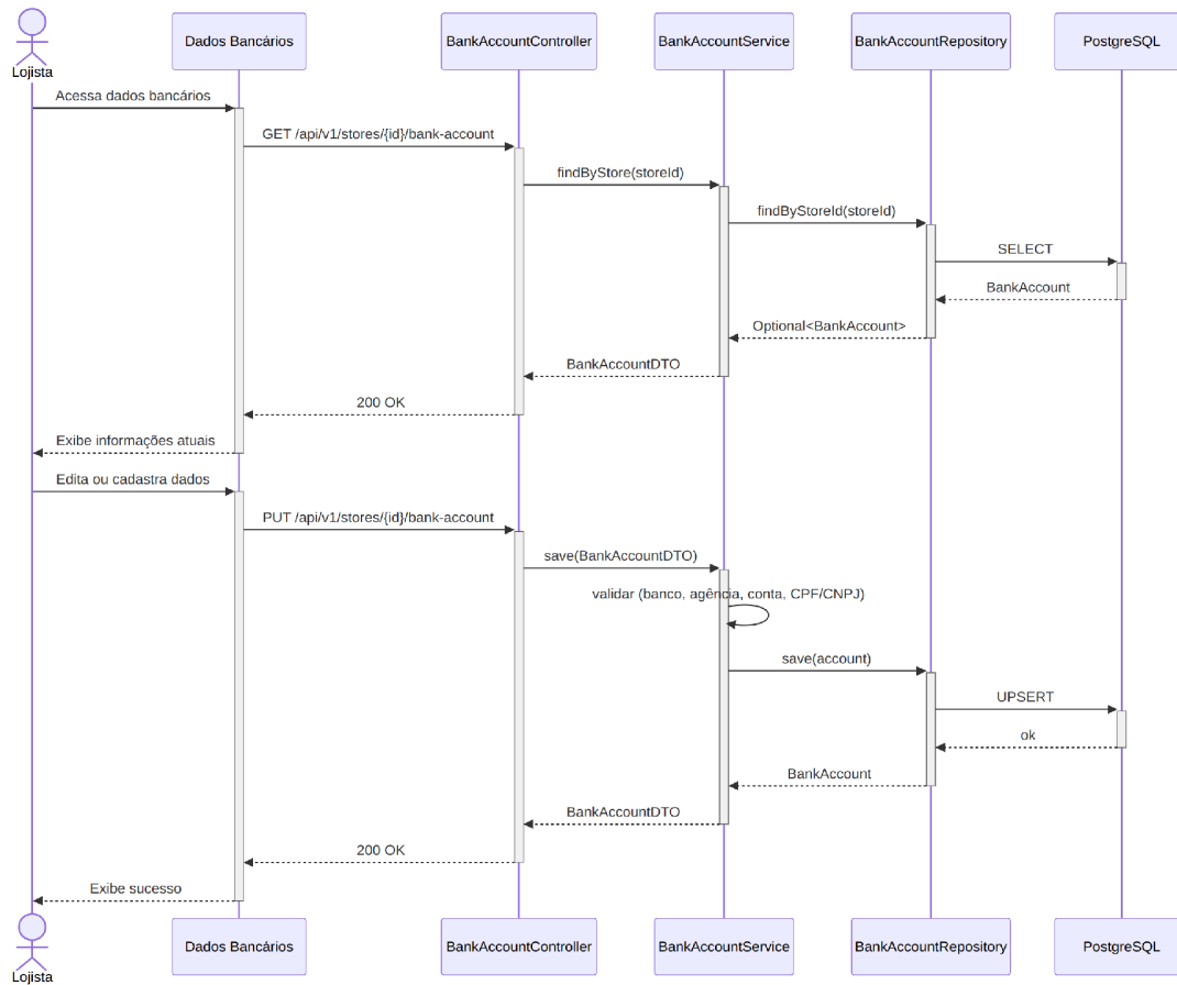
Figura 12 — Diagrama de sequência do UC12 (Gerenciar dados bancários).
