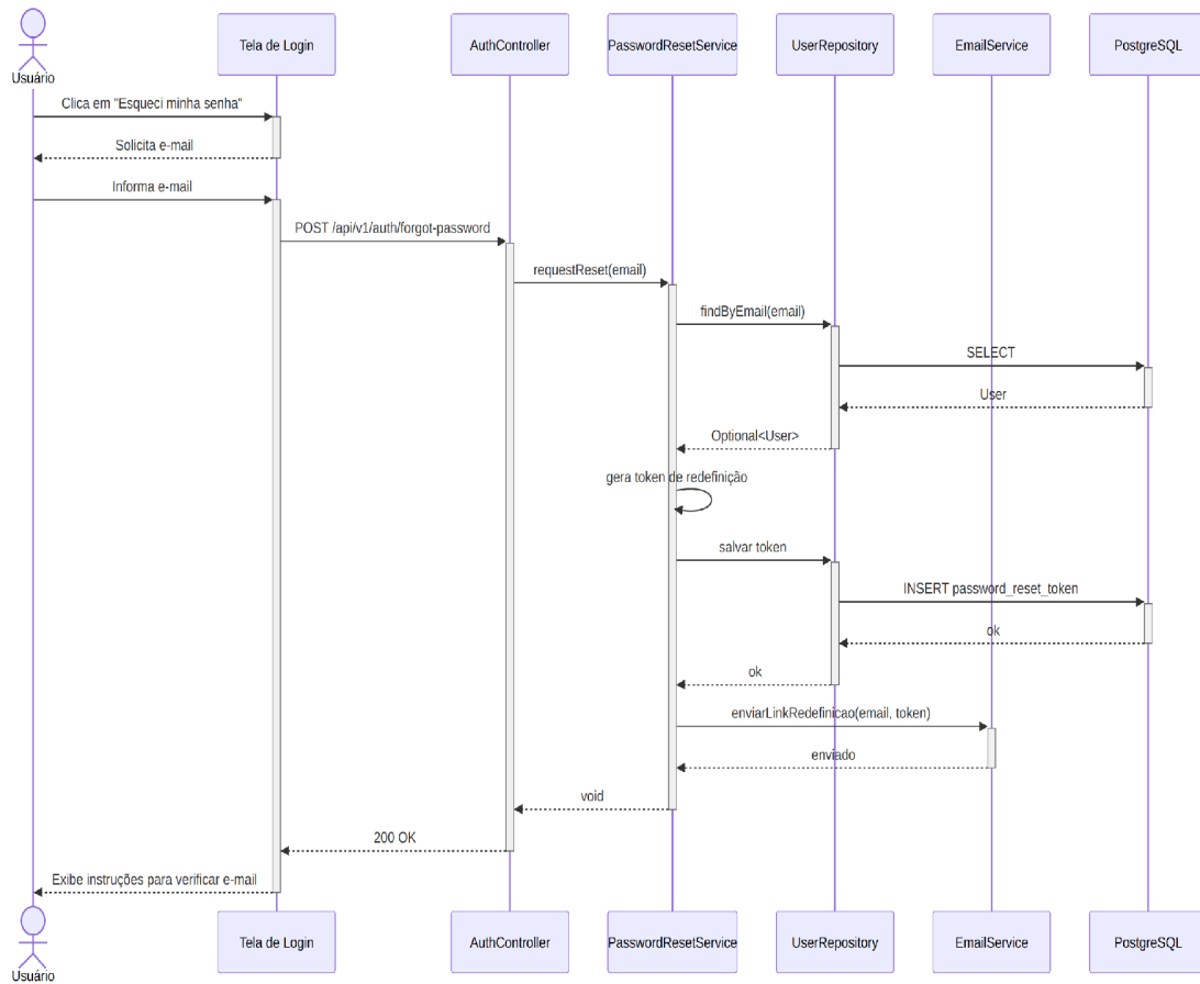
Figura 3 — Diagrama de sequência do UC03 (Recuperar senha).
