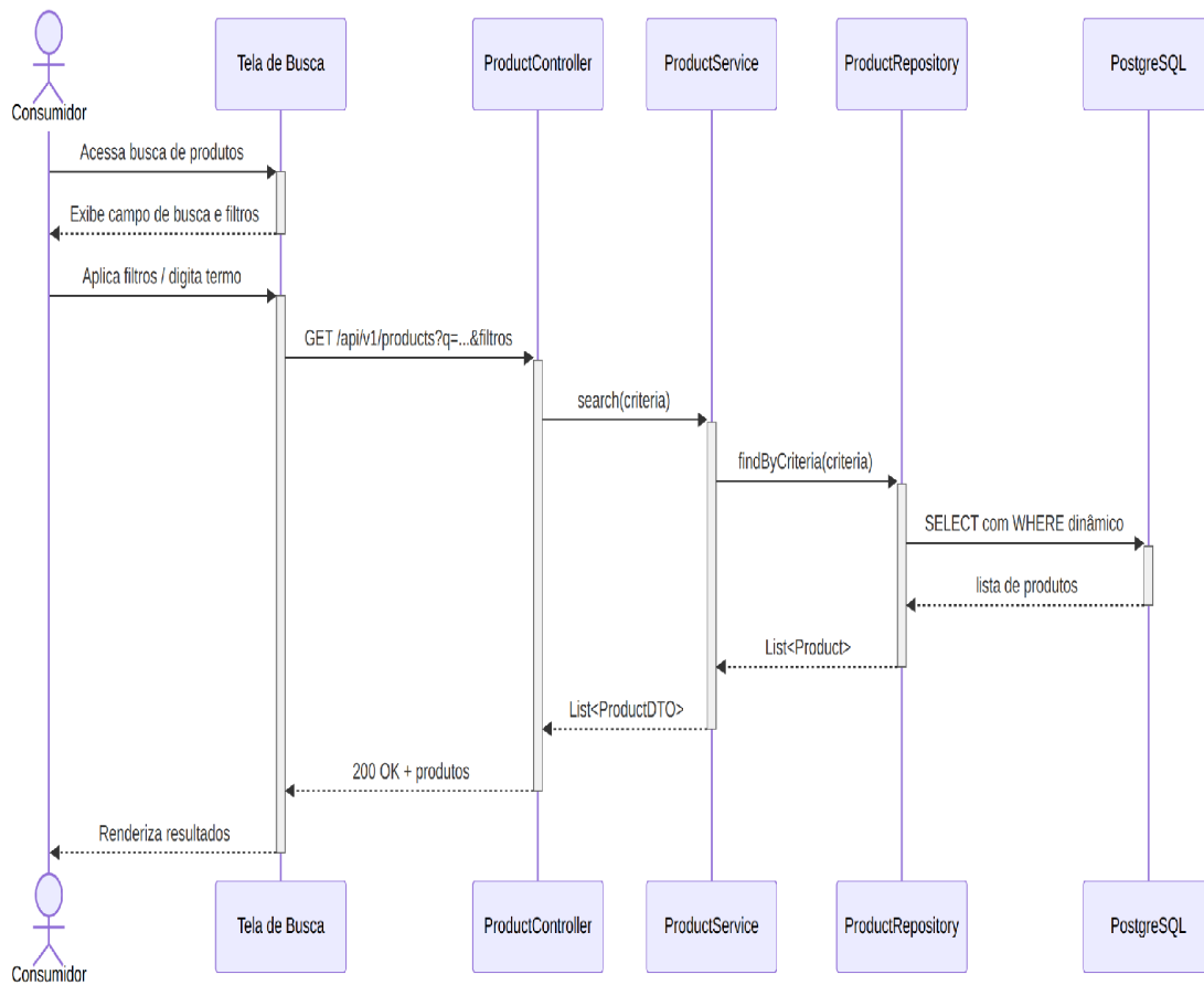
Figura 4 — Diagrama de sequência do UC04 (Buscar e filtrar produtos).
