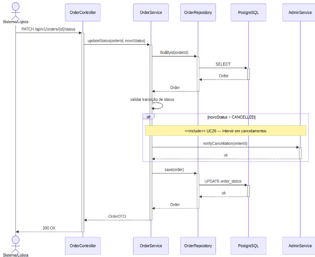
Figura 15 — Diagrama de sequência do UC15 (Atualizar status do pedido).
