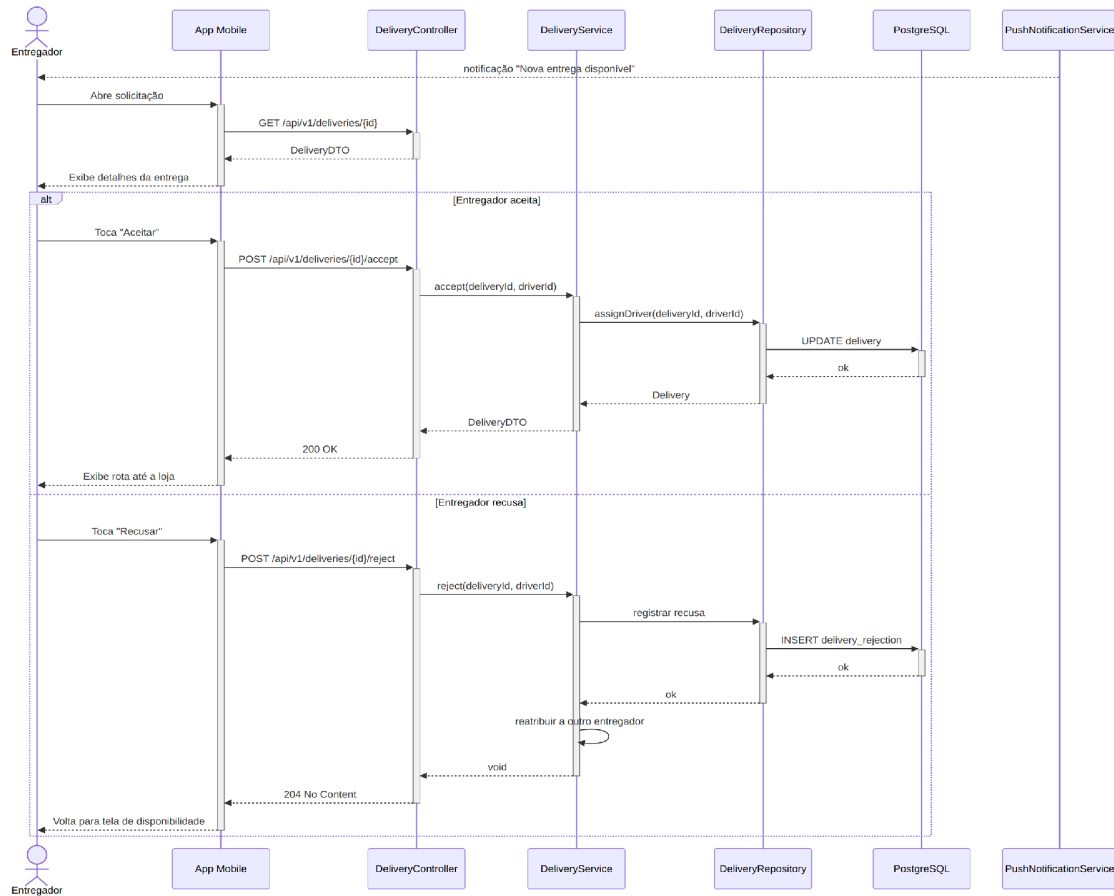
Figura 19 — Diagrama de sequência do UC19 (Aceitar ou recusar entrega).
