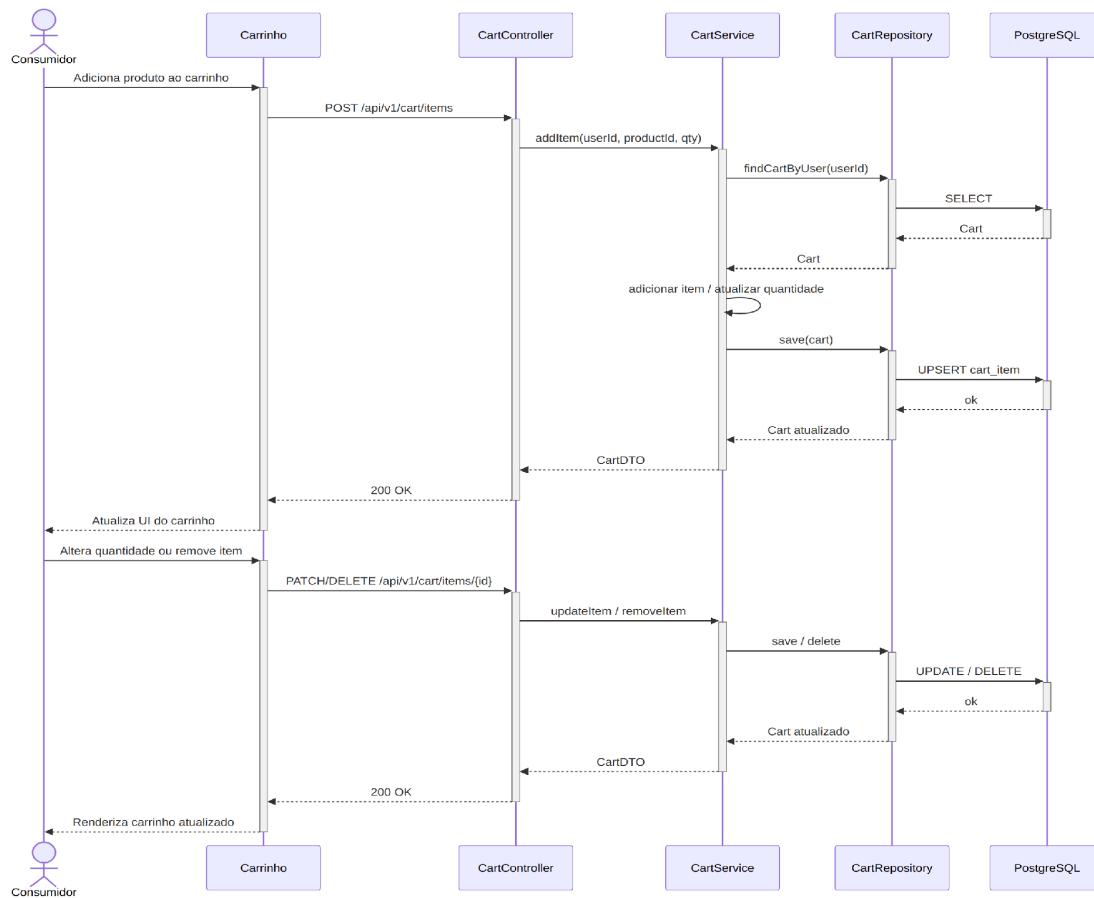
Figura 6 — Diagrama de sequência do UC06 (Gerenciar carrinho).
