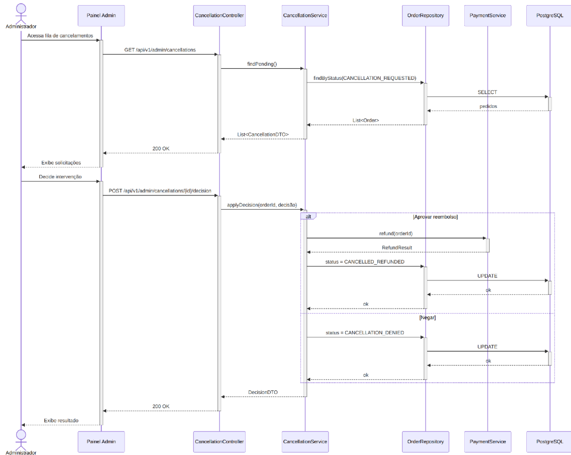
Figura 26 — Diagrama de sequência do UC26 (Intervir em cancelamentos).
