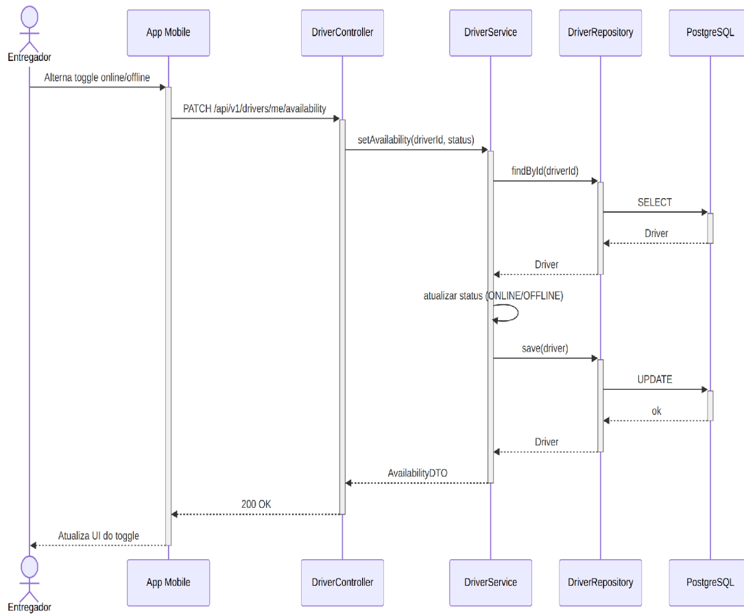
Figura 18 — Diagrama de sequência do UC18 (Alternar disponibilidade online/offline).
