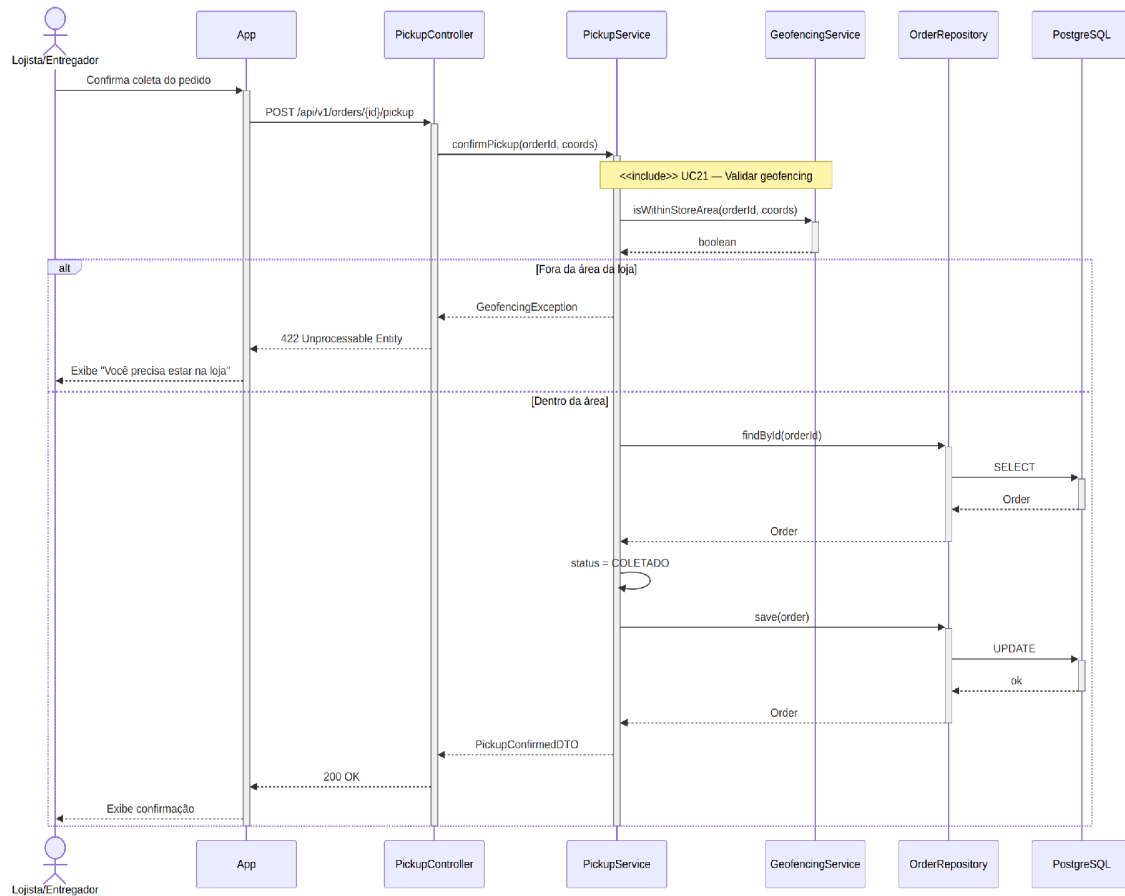
Figura 14 — Diagrama de sequência do UC14 (Confirmar coleta na loja).
