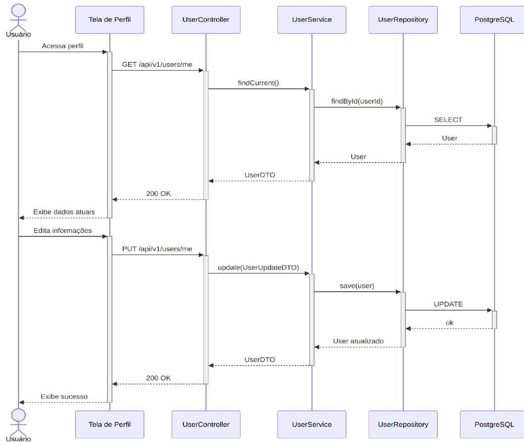
Figura 10 — Diagrama de sequência do UC10 (Gerenciar perfil).
