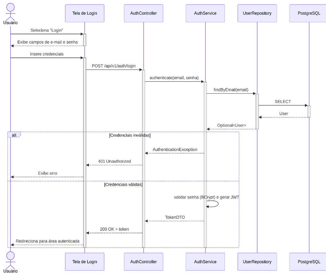
Figura 2 — Diagrama de sequência do UC02 (Fazer login).
