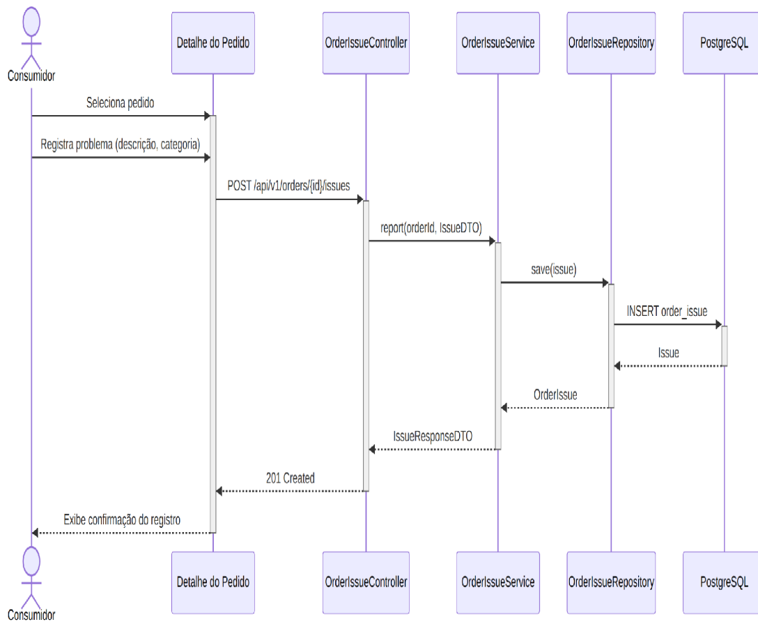
Figura 9 — Diagrama de sequência do UC09 (Relatar problema na entrega).
