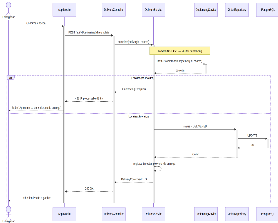
Figura 20 — Diagrama de sequência do UC20 (Confirmar entrega ao consumidor).
