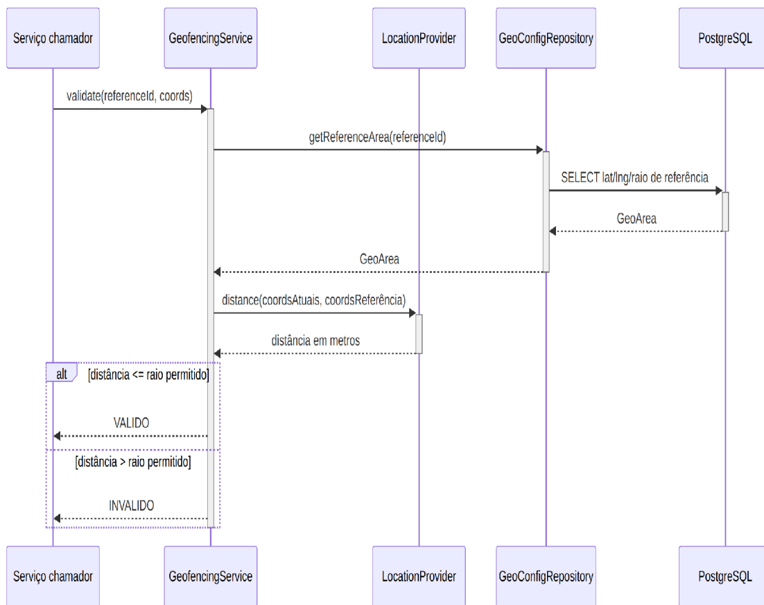
Figura 21 — Diagrama de sequência do UC21 (Validar geofencing).
