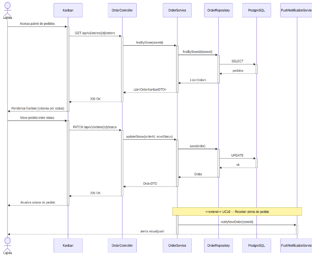
Figura 13 — Diagrama de sequência do UC13 (Gerenciar pedidos (Kanban)).
