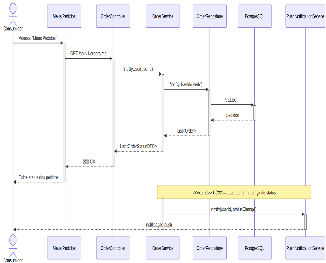
Figura 8 — Diagrama de sequência do UC08 (Acompanhar pedido).
