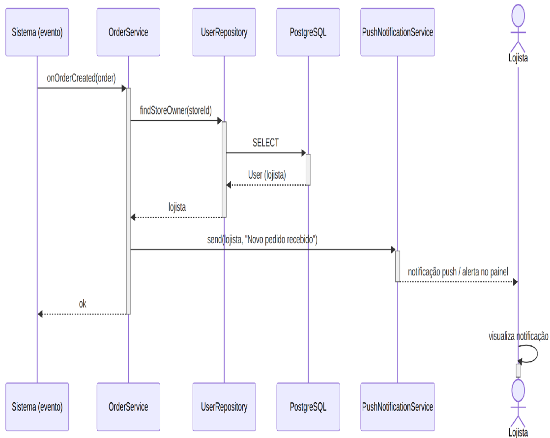
Figura 16 — Diagrama de sequência do UC16 (Receber alerta de pedido).
