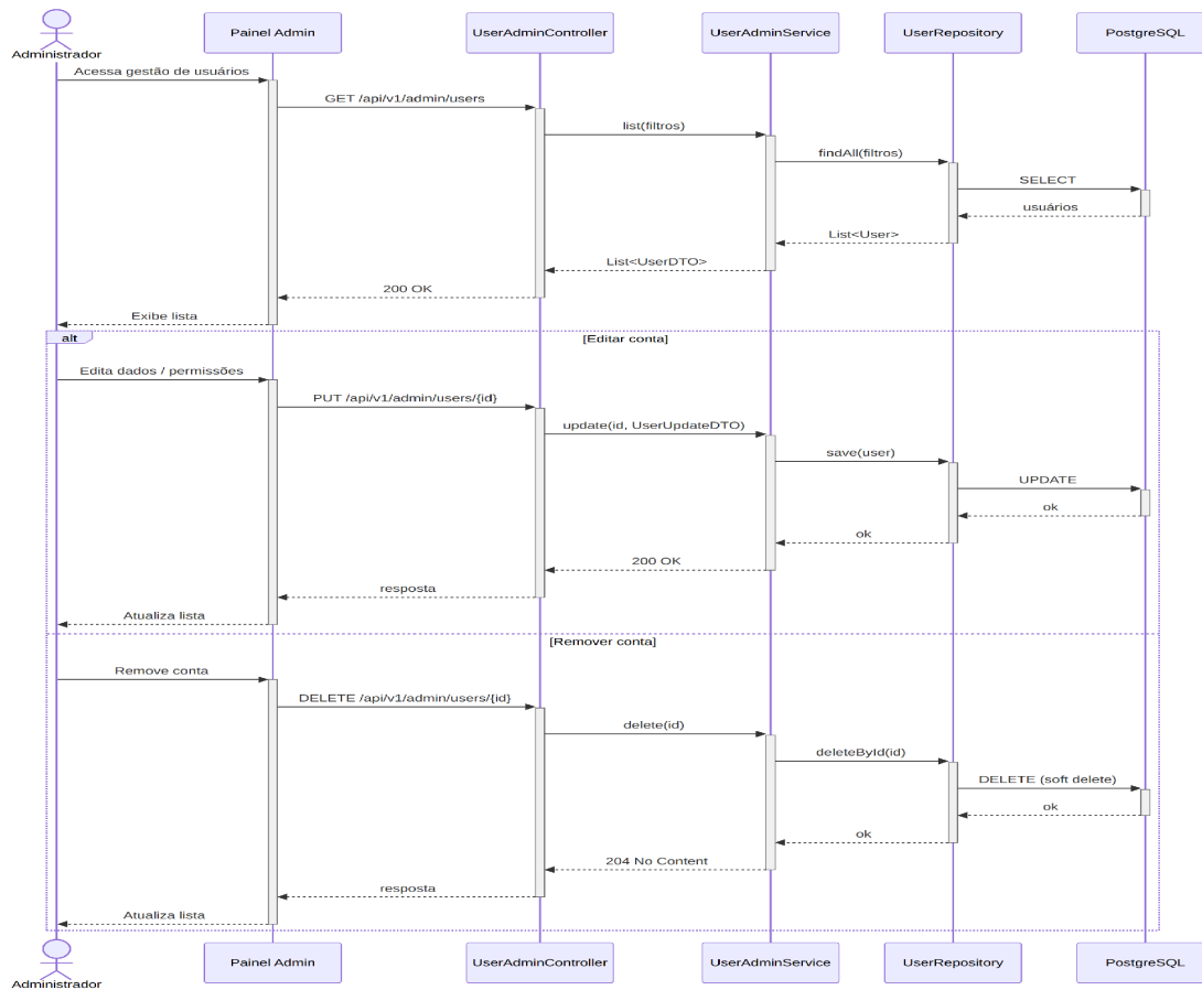
Figura 25 — Diagrama de sequência do UC25 (Gerenciar contas de usuários).
