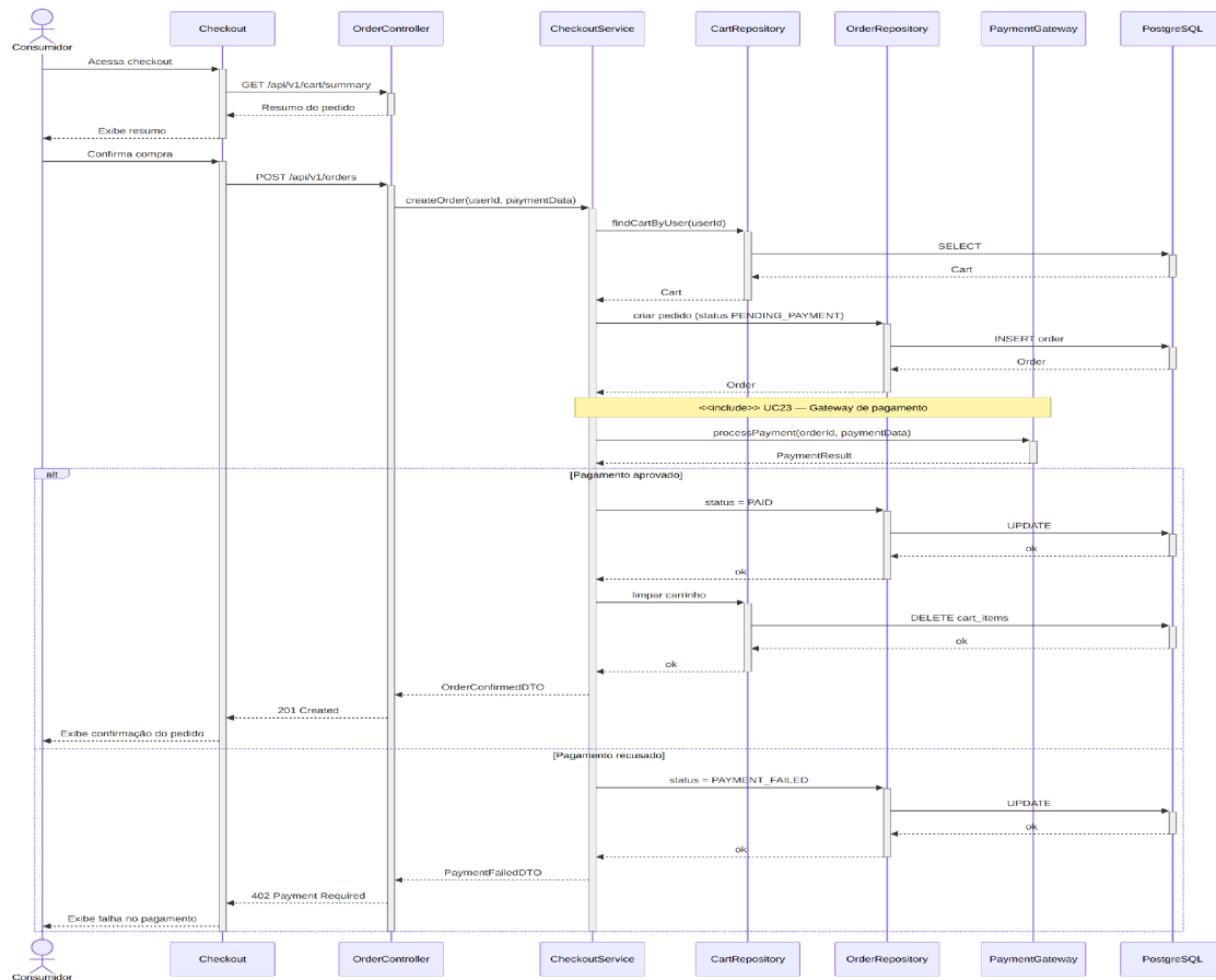
Figura 7 — Diagrama de sequência do UC07 (Realizar checkout).
