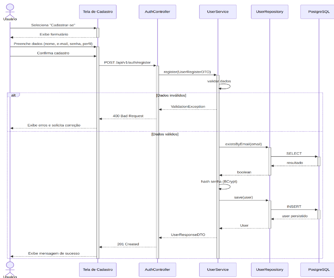
Figura 1 — Diagrama de sequência do UC01 (Cadastrar-se na plataforma).
