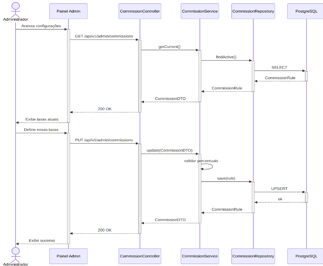
Figura 17 — Diagrama de sequência do UC17 (Configurar taxas de comissão).
